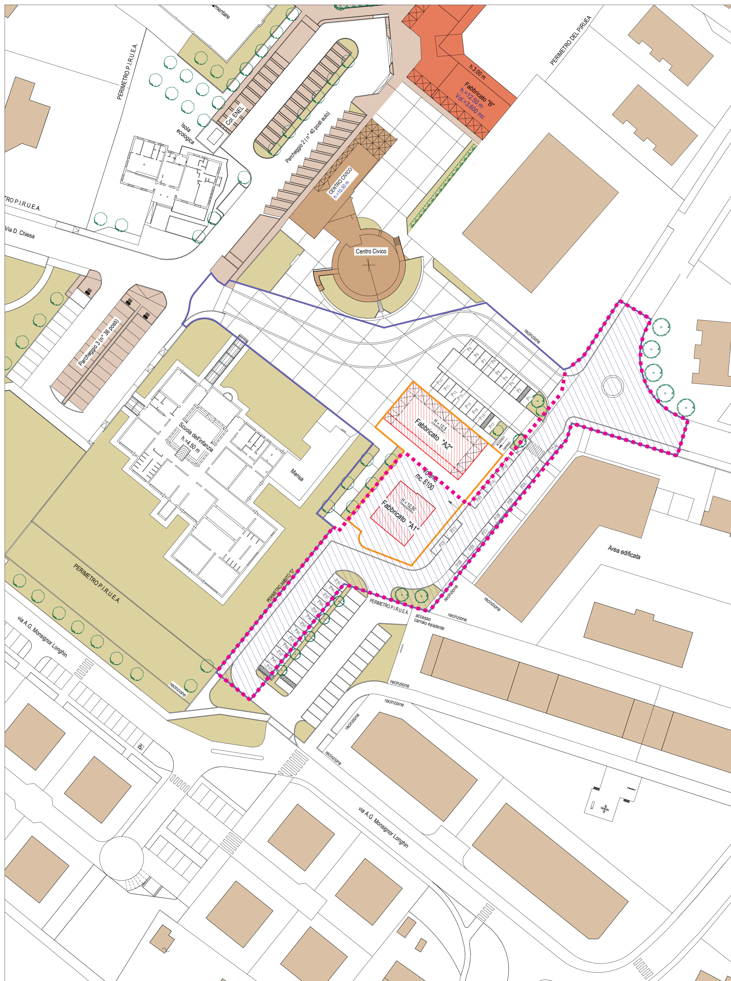
PLANIMETRIA CON INDIVIDUAZIONE STRALCI OPERE DI URBANIZZAZIONE COMPARTO "D"
