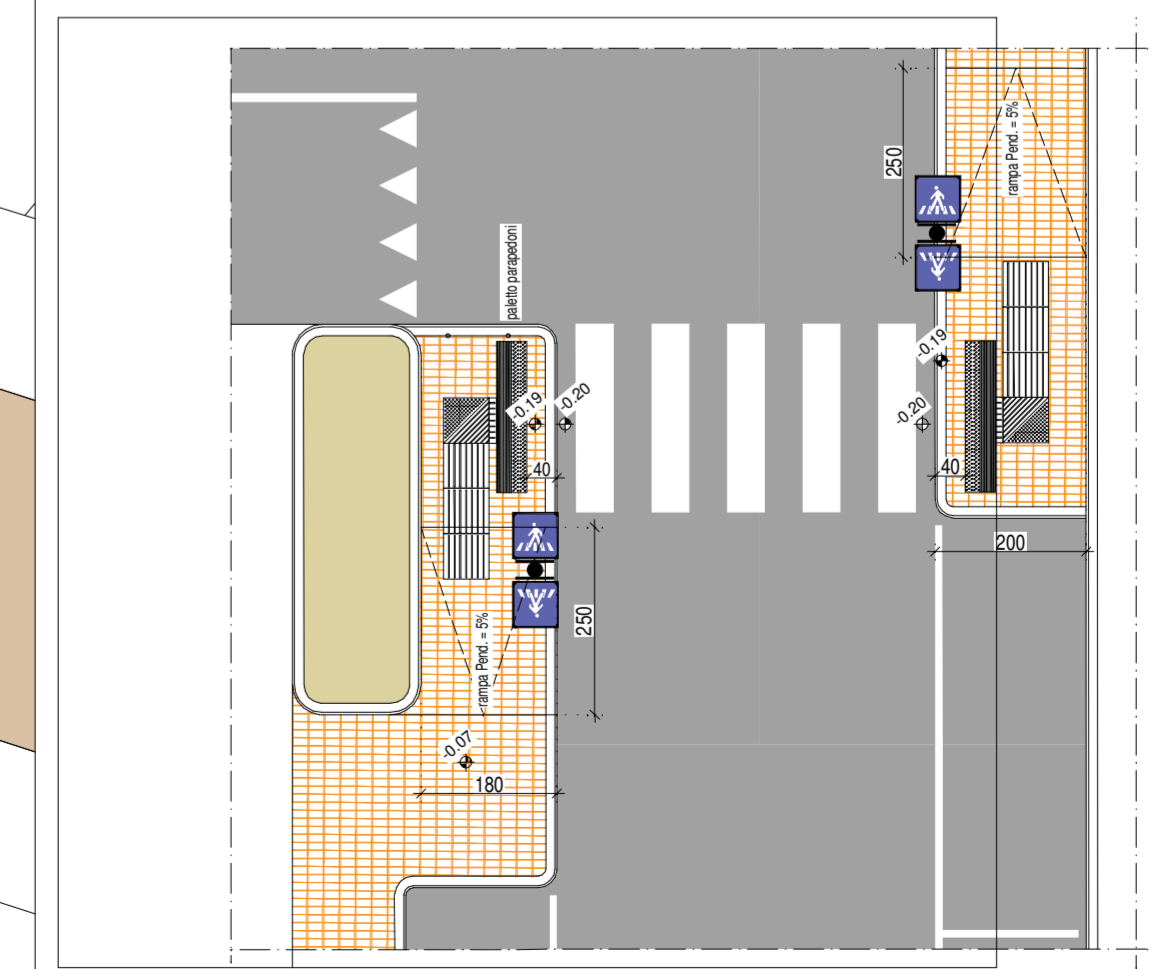
PARTICOLARE ATTRAVERSAMENTO PEDONALE SCALA 1:100
