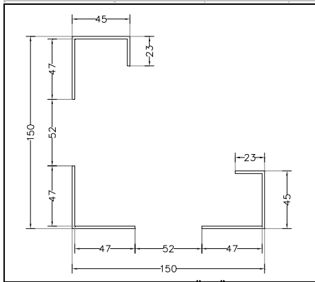
SEZIONE EFFICACE
