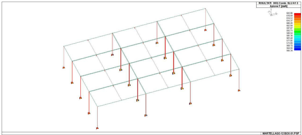
42_RIS_REAZIONI_003_Comb. SLU A1 3
