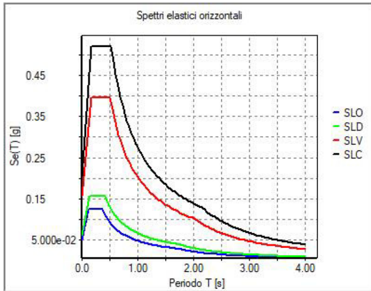
01_INT_SPETTRI_ELASTICI_O
