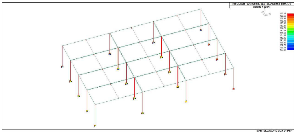
42_RIS_REAZIONI_076_Comb. SLE (SLD Danno sism.) 76
