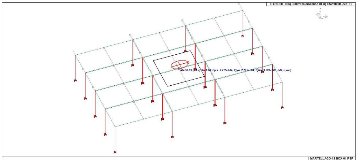
22_CDC_006_CDC=Ed (dinamico SLU) alfa=90.00 (ecc. +)
