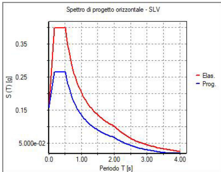
31_RIS_SPETTRI_PROGETTO_SLV_O
