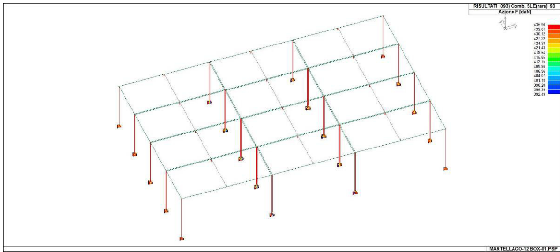
42_RIS_REAZIONI_093_Comb. SLE(rara) 93
