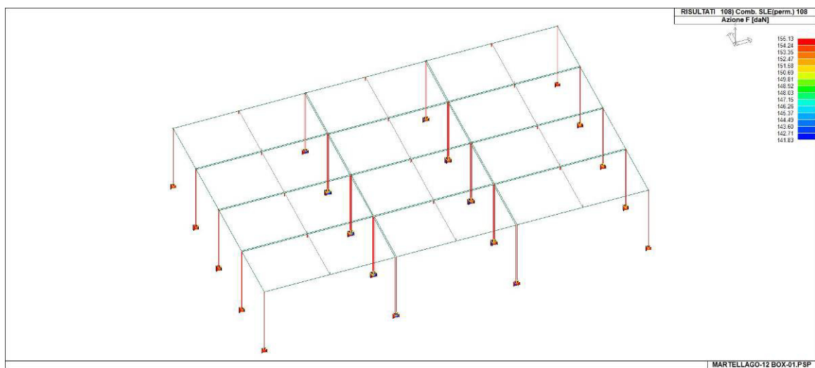
42_RIS_REAZIONI_108_Comb. SLE(perm.) 108
