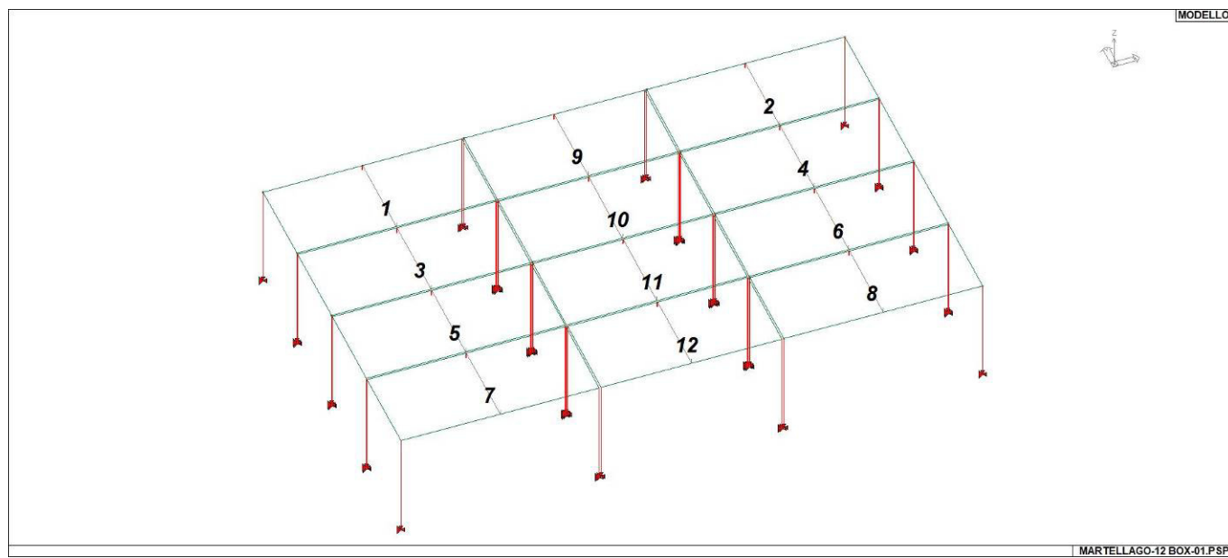
17_MOD_NUMERAZIONE_SOLAI
