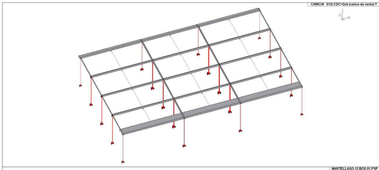
22_CDC_013_CDC=Qvk (carico da vento) Y
