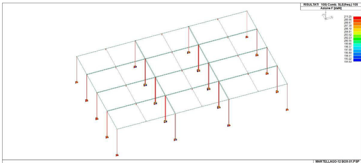
42_RIS_REAZIONI_105_Comb. SLE(freq.) 105
