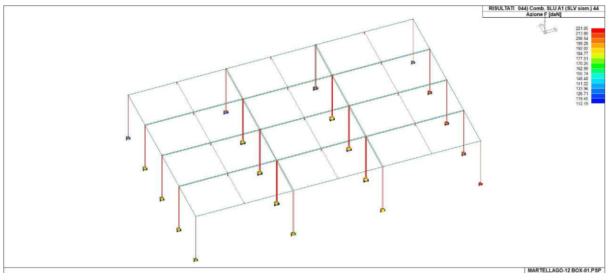
42_RIS_REAZIONI_044_Comb. SLU A1 (SLV sism.) 44
