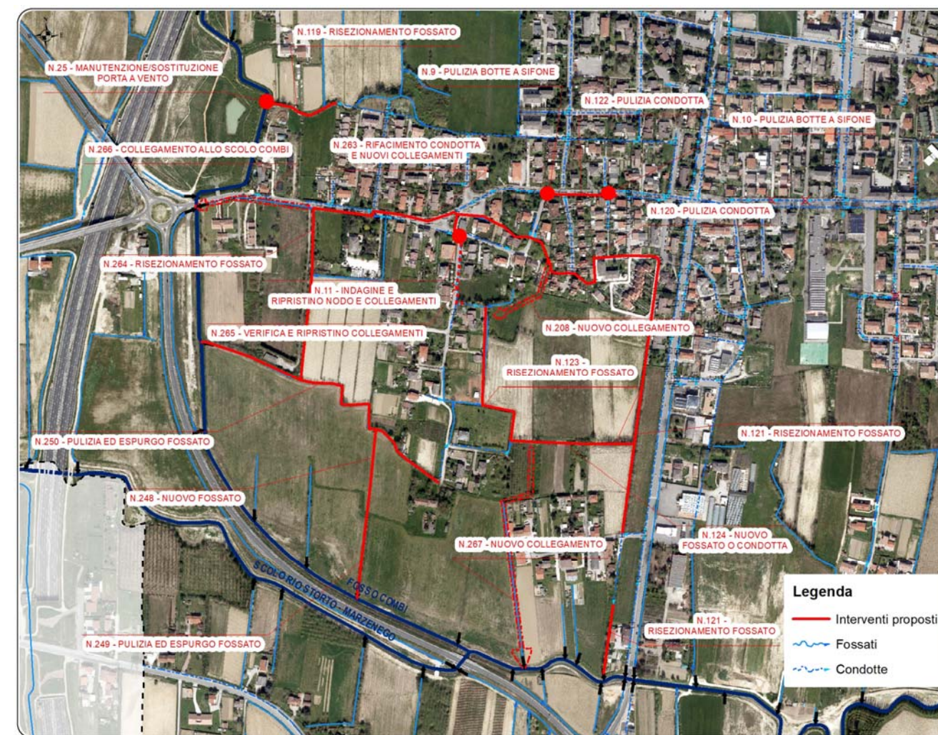
Planimetria ipotesi di intervento
