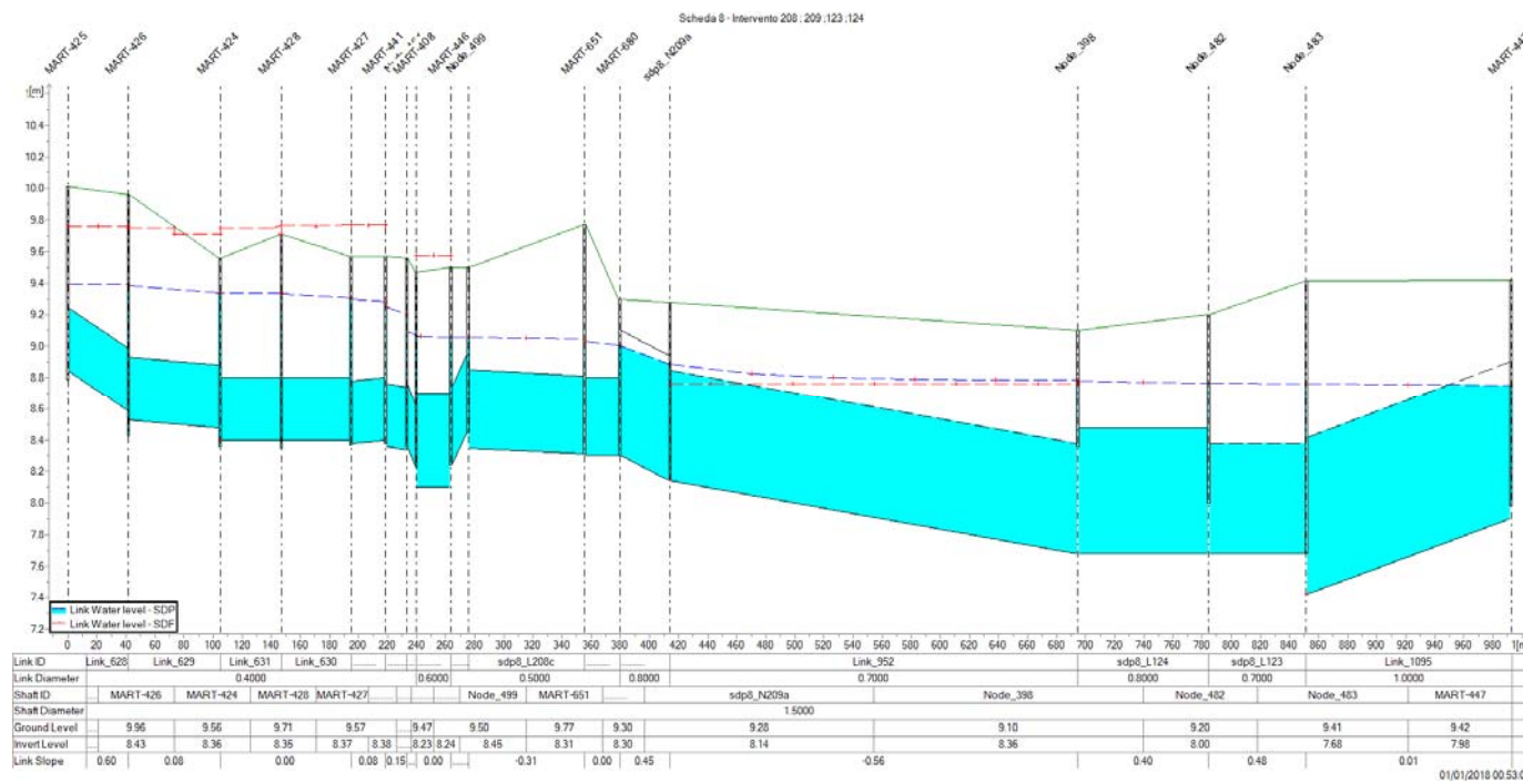
Profilo del tombinamento via Motte e suo scarico (rosso= stato di fatto, blu= stato di progetto)
