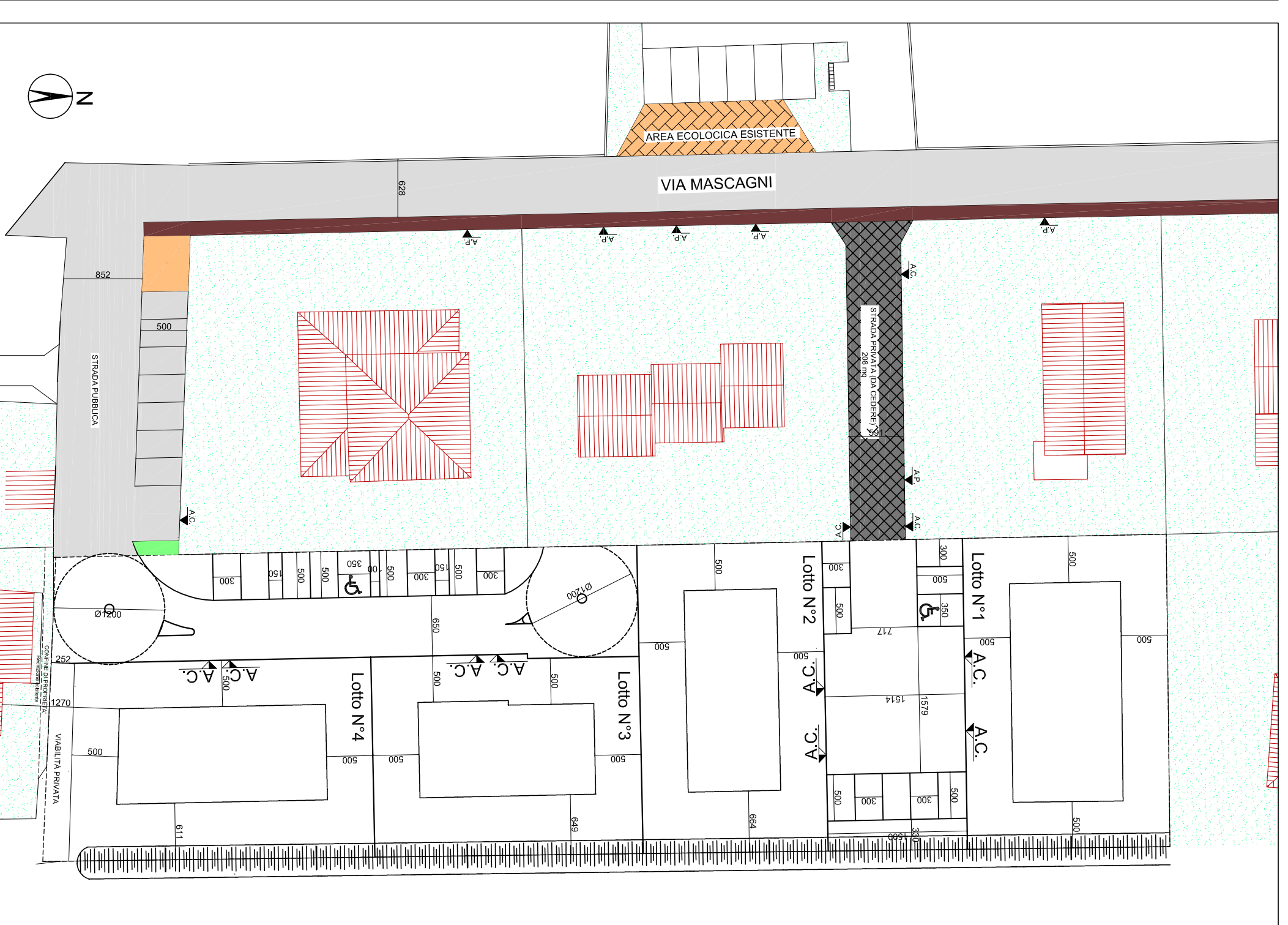
PLANIMETRIA DI DIMENSIONAMENTO Scala 1:500
