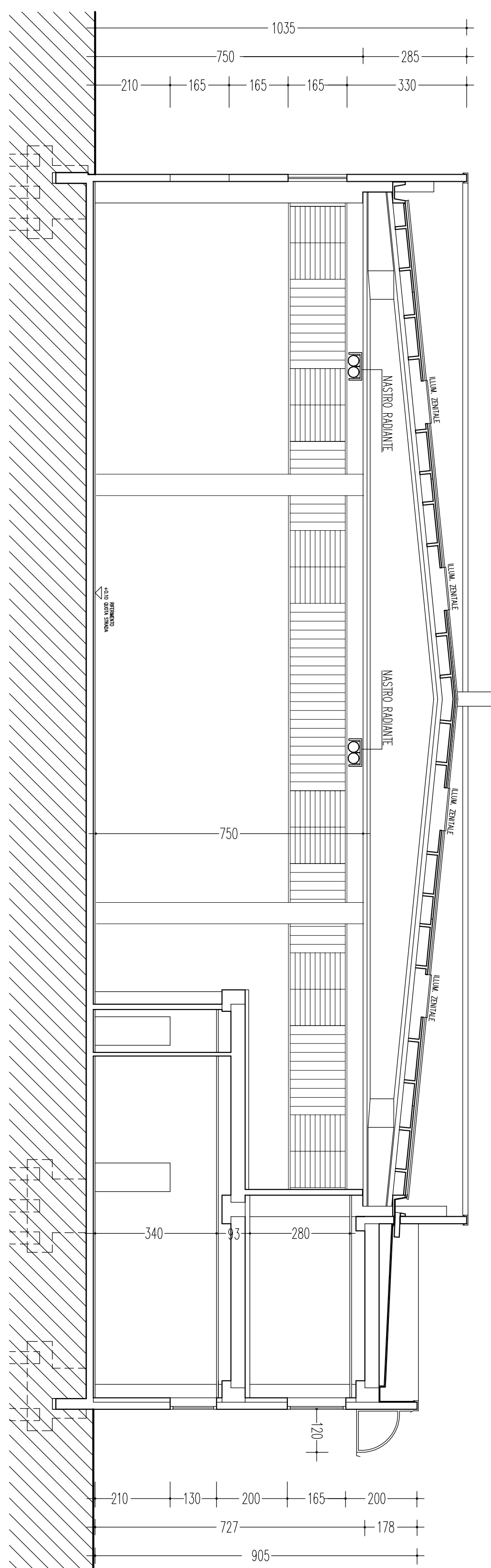
SEZIONE D-D scala 1/100
