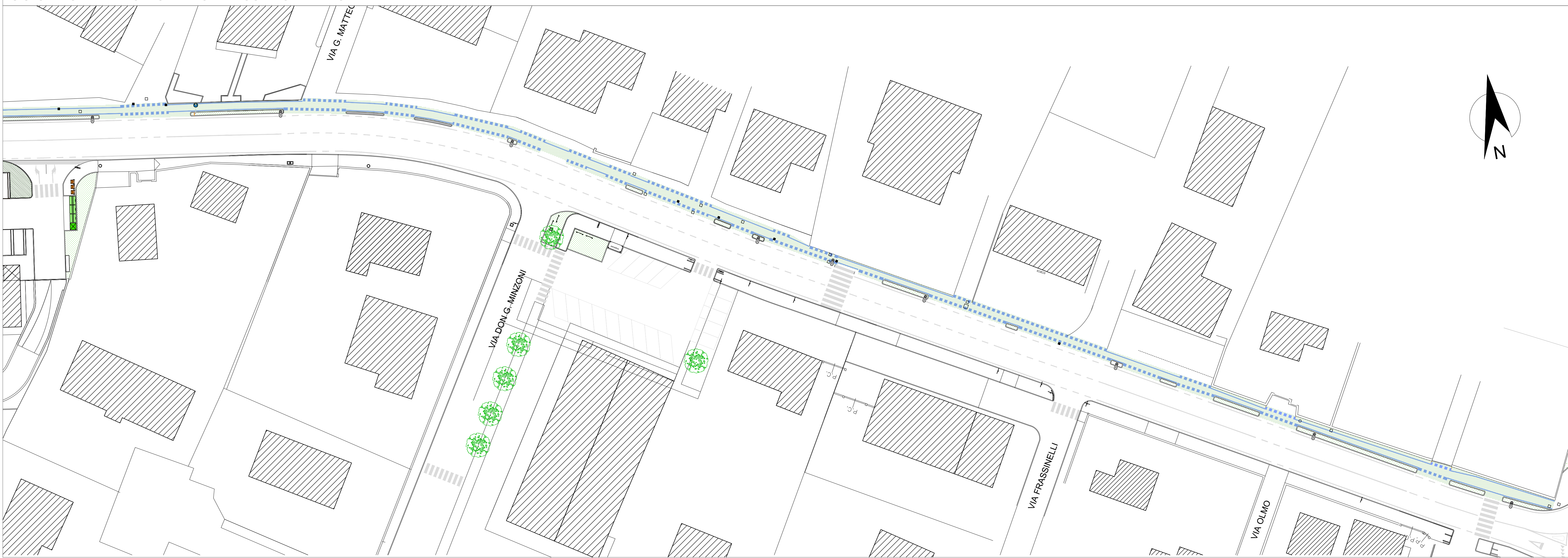
CICLOPEDONALE VIA OLMO: STATO DI PROGETTO - TRATTO 4
