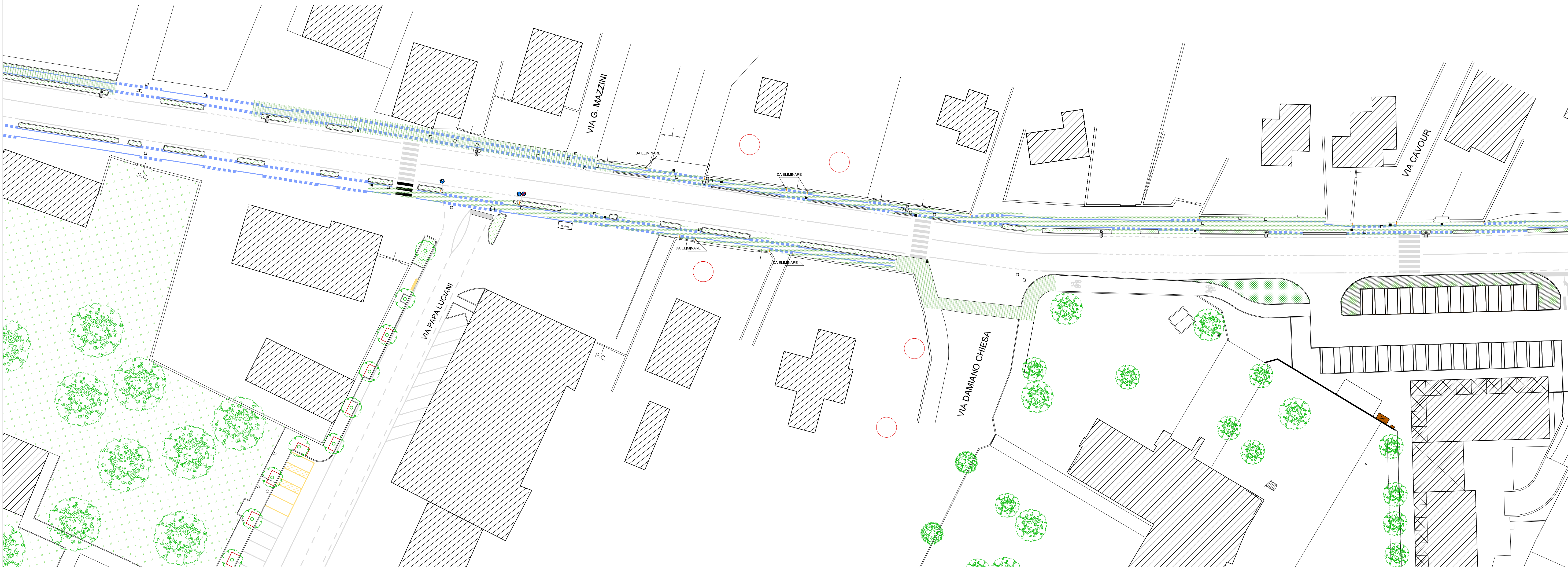
CICLOPEDONALE VIA OLMO: STATO DI PROGETTO - TRATTO 4
