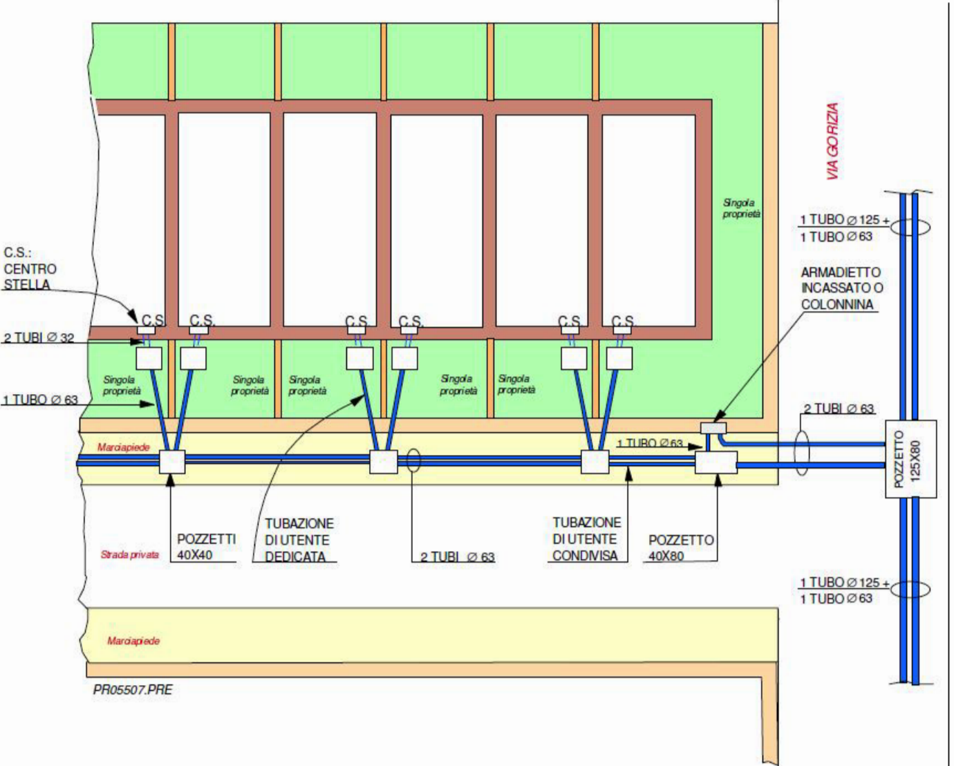
Figura A. 9 - Esempio di predisposizione per case a schiera con armadietto o colonnina
